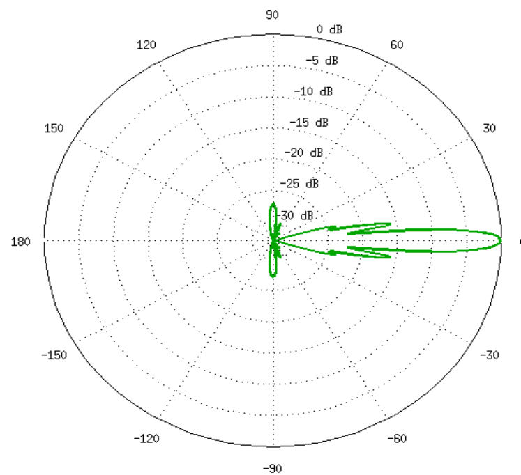
H-Plane 5.5GHz
