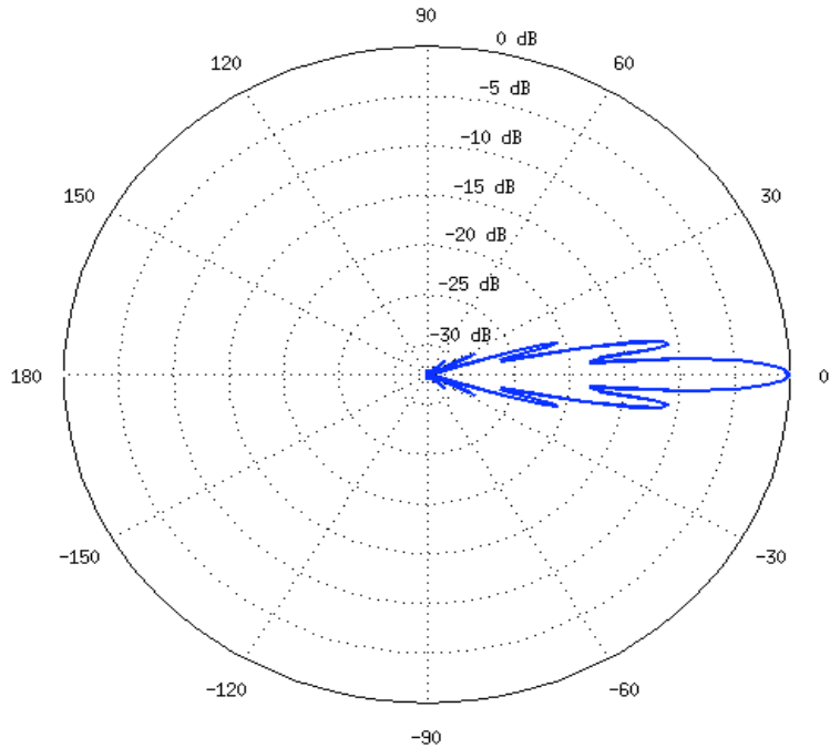
E-Plane, 5.5GHz
